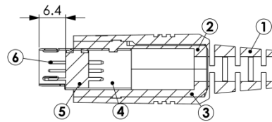
A-A SECTION
